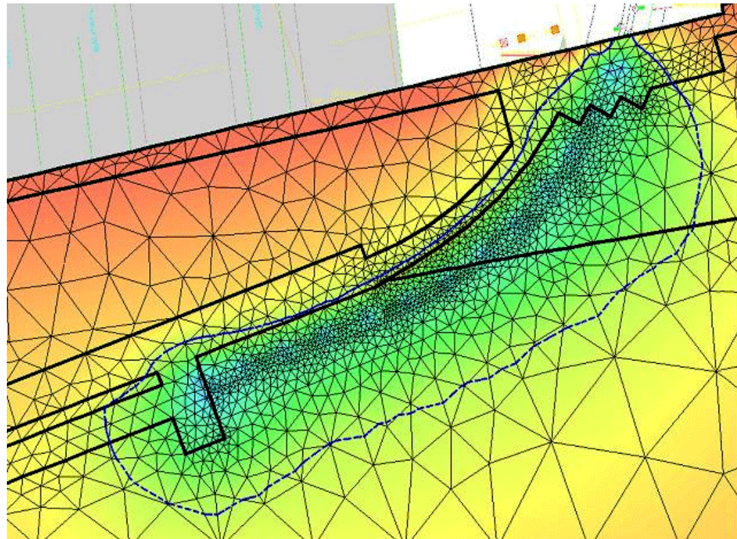
Een overzicht van het temperatuur verloop tijdens de instandhoud fase met in blauw -35 graden Celsius en in rood +20 graden Celsius. De blauwe lijn geeft de 0 graden grens.
