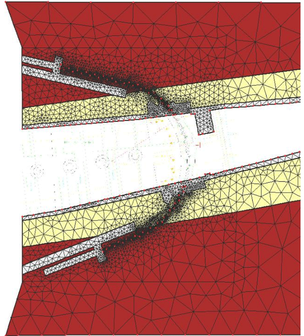
Een bovenaanzicht van een doorsnede met in bruin veen, in geel zand, in grijs beton en in het midden de metrobus.
