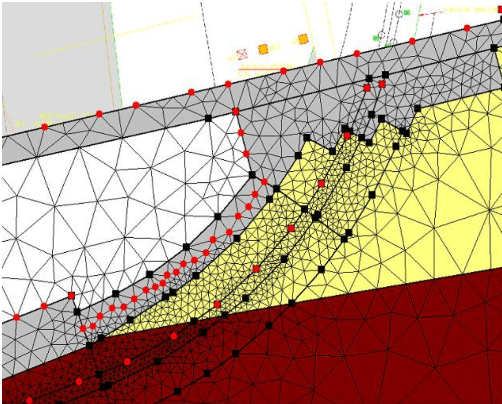
Een detail van het model bij een ontgraving (de witte cellen), het uitharden van het beton (hydratatiewarmte op het vrieslichaam) en het instandhouden van de kraagconstructie
